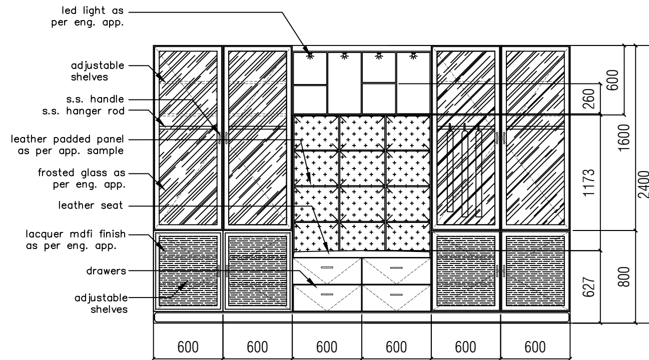
ELEVATION
